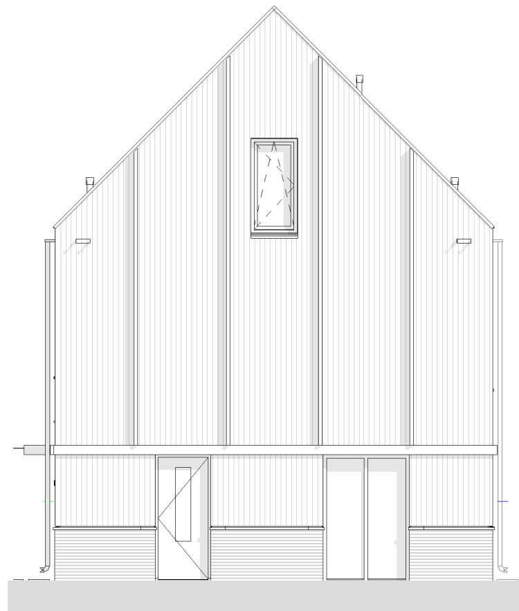
zijgevel (oost)
