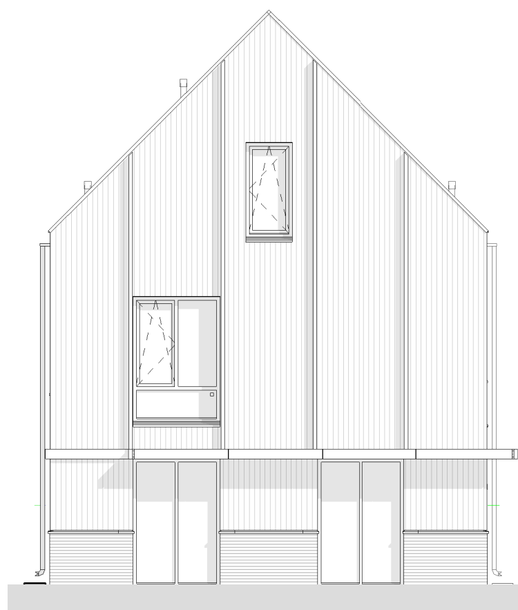
zijgevel (west)
