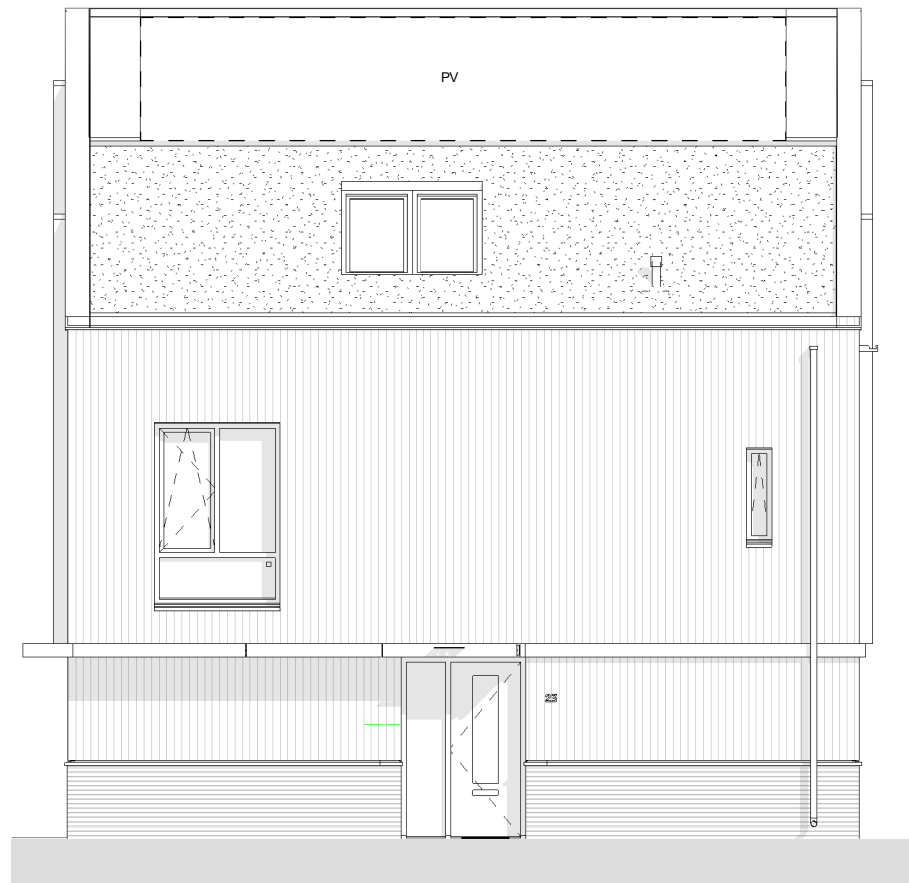
voorgevel (zuid)
